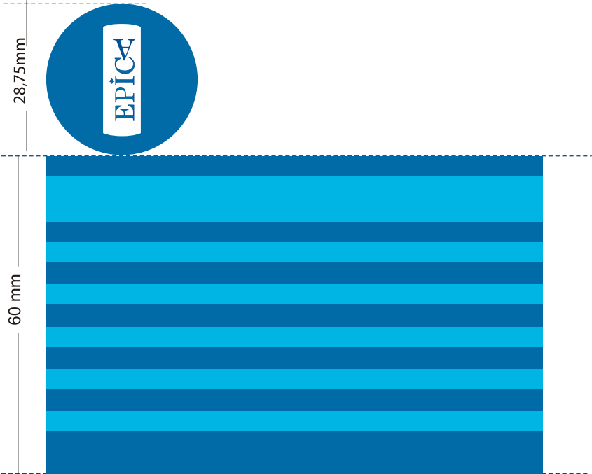
Desarrollo Plano
