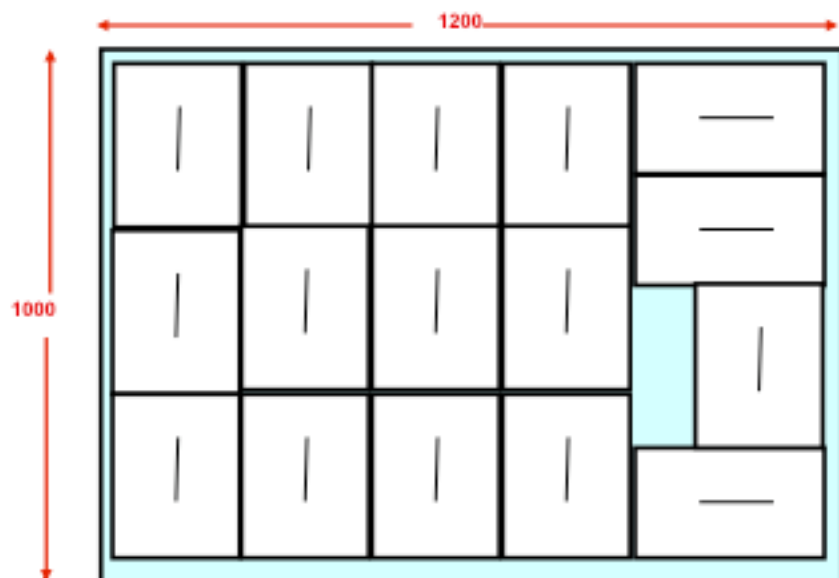
CAMADA 1 (16 Cajas)
