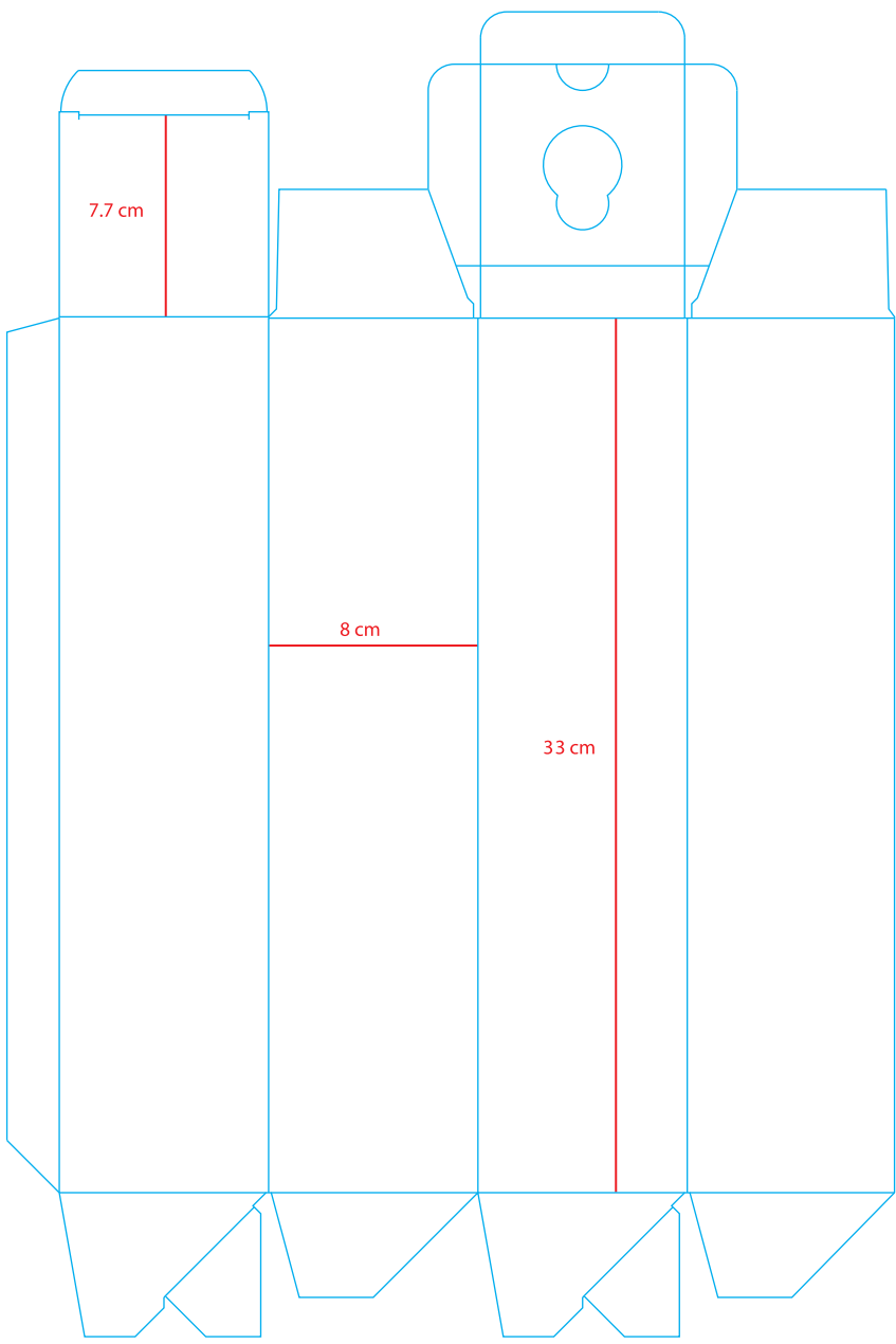
TROQUEL
