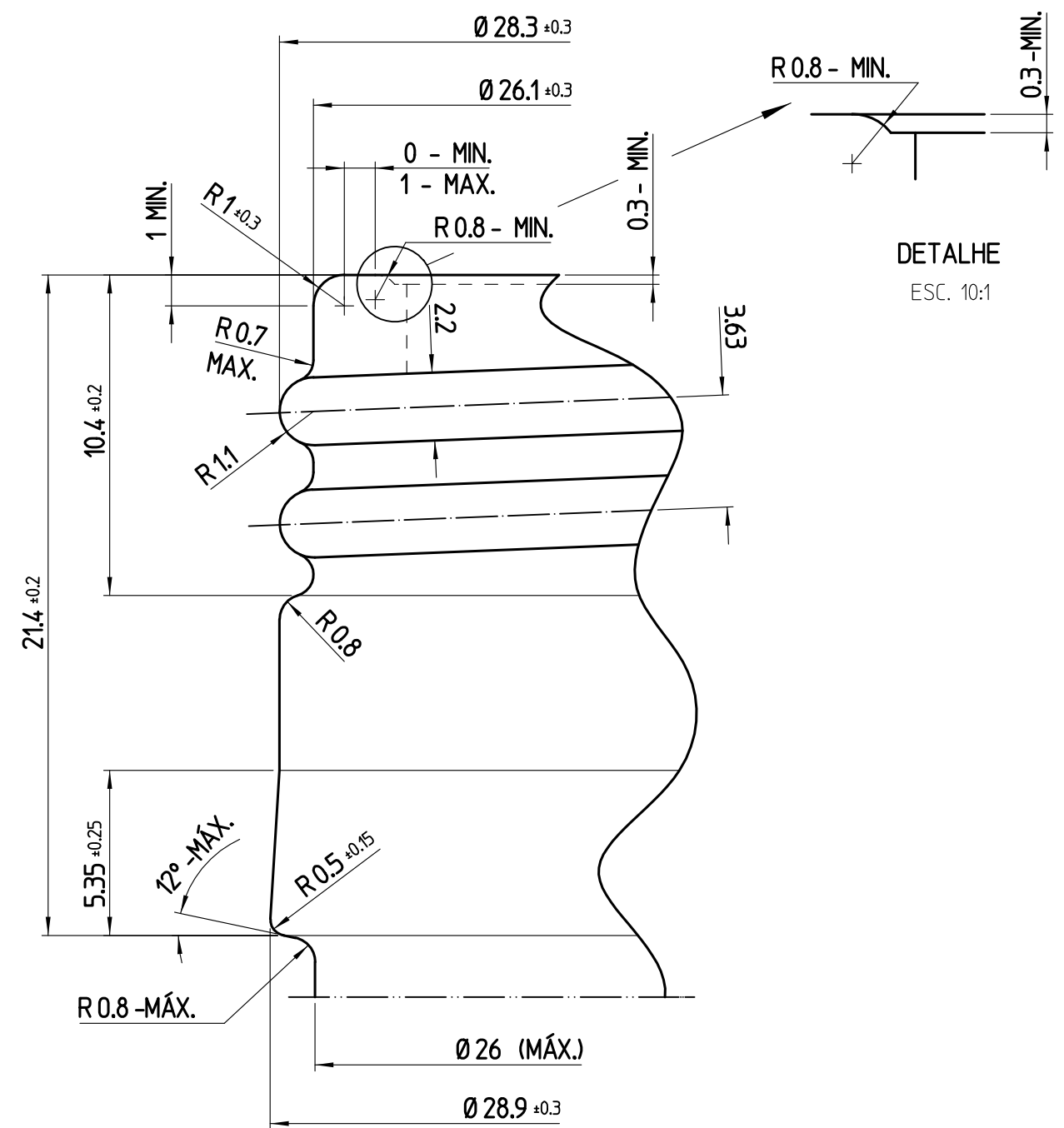
CORTE A-A ESC. 5:1
