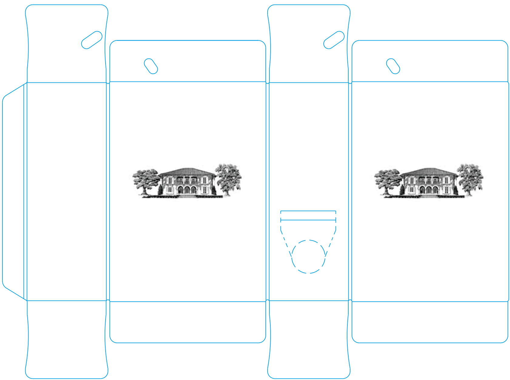
Aplicación Sobreimpresión Folia Oro Esc. 40%
