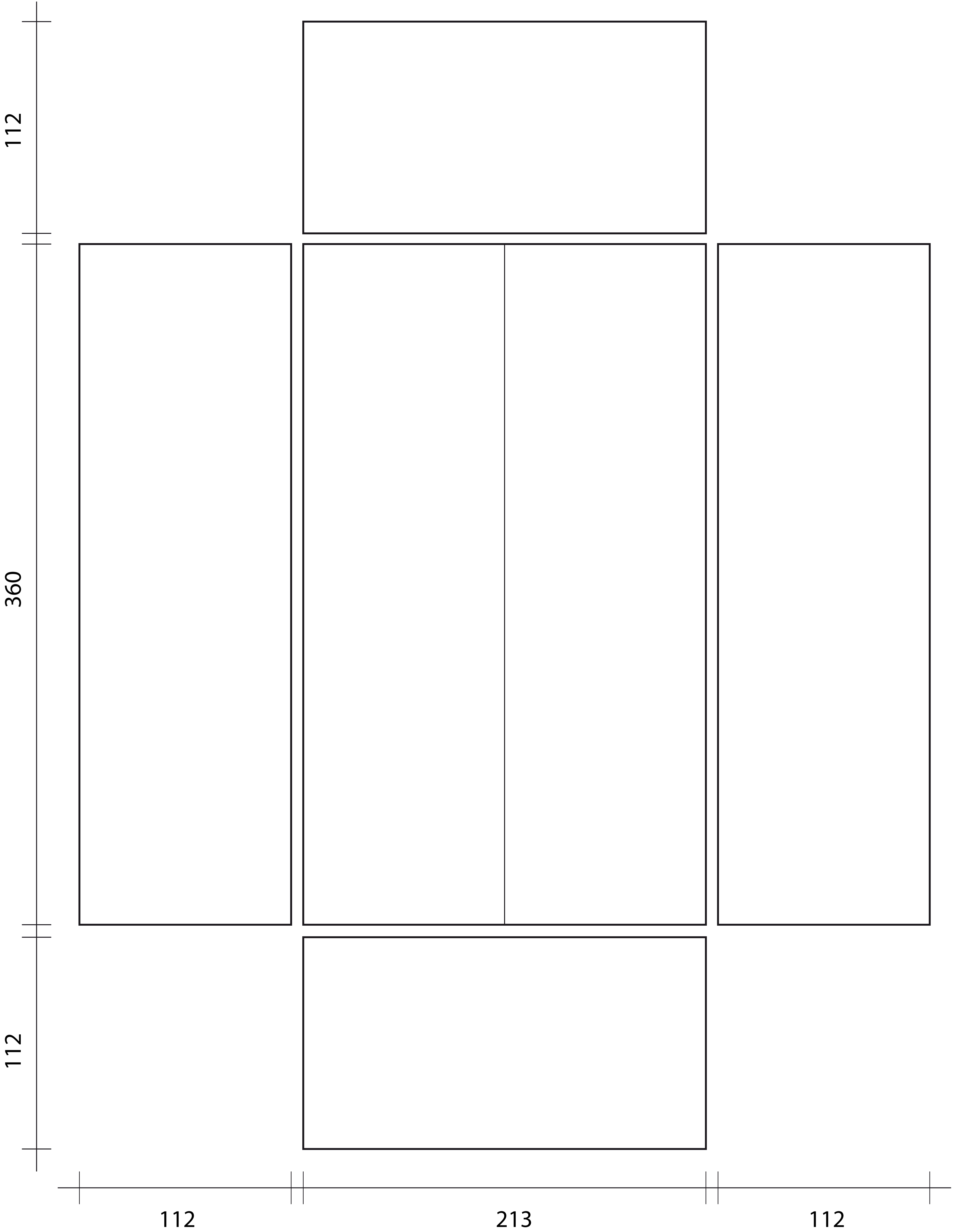
Vista posterior en despiece - Medidas generales Esc 1:1 (Medidas en mm.)
