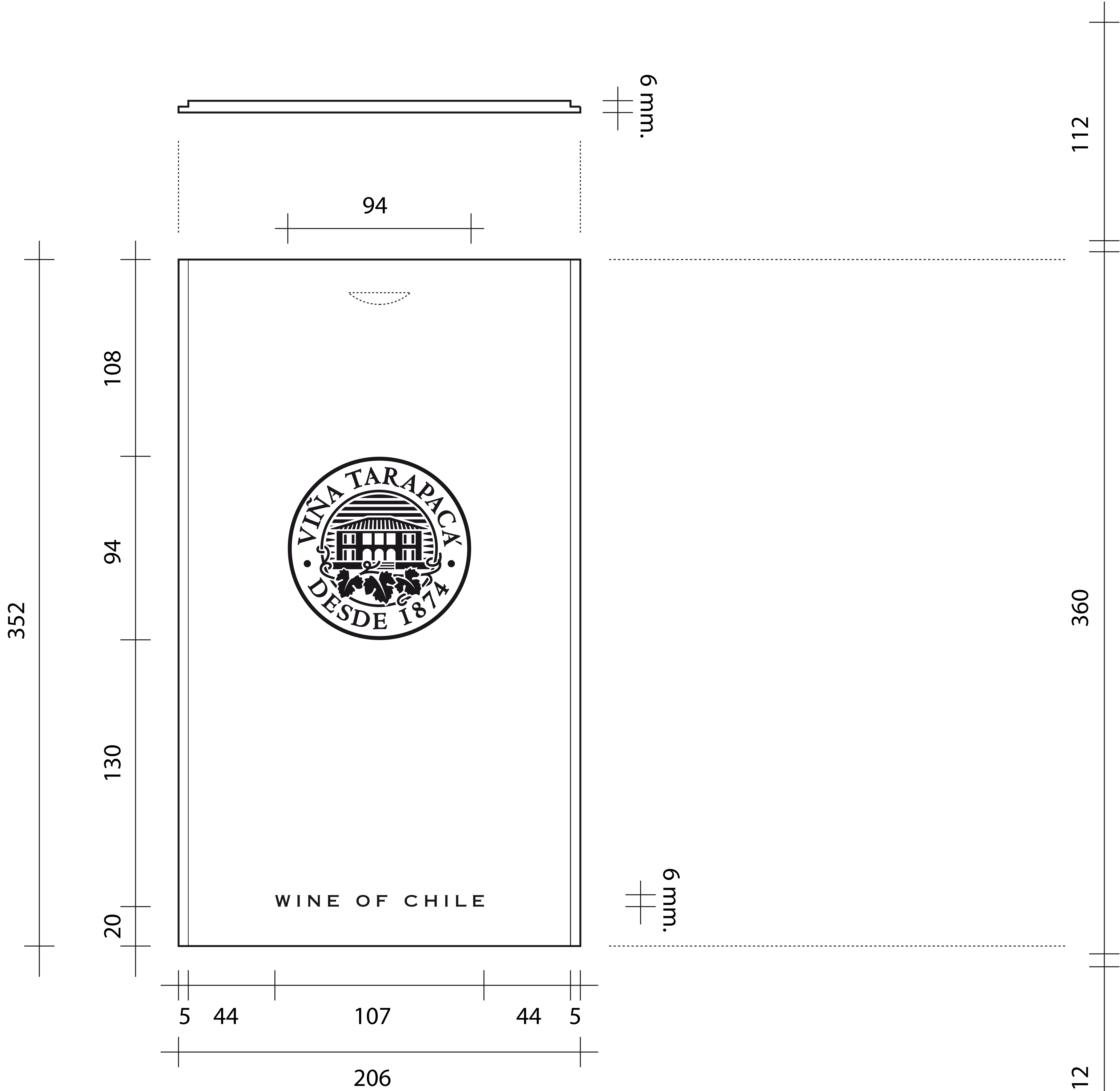
Vista frontal Tapa Esc 1:1 (Medidas en mm.)
