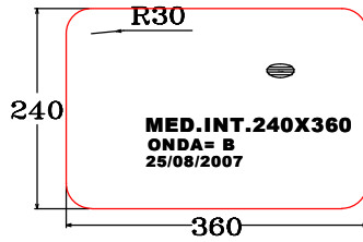
CAD PARA MATRIZ Y HOJA CORRUGADA (12 SET)
