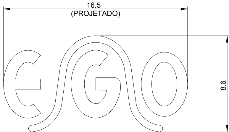
DETALHE DA GRAVAÇÃO ESCALA 5:1
