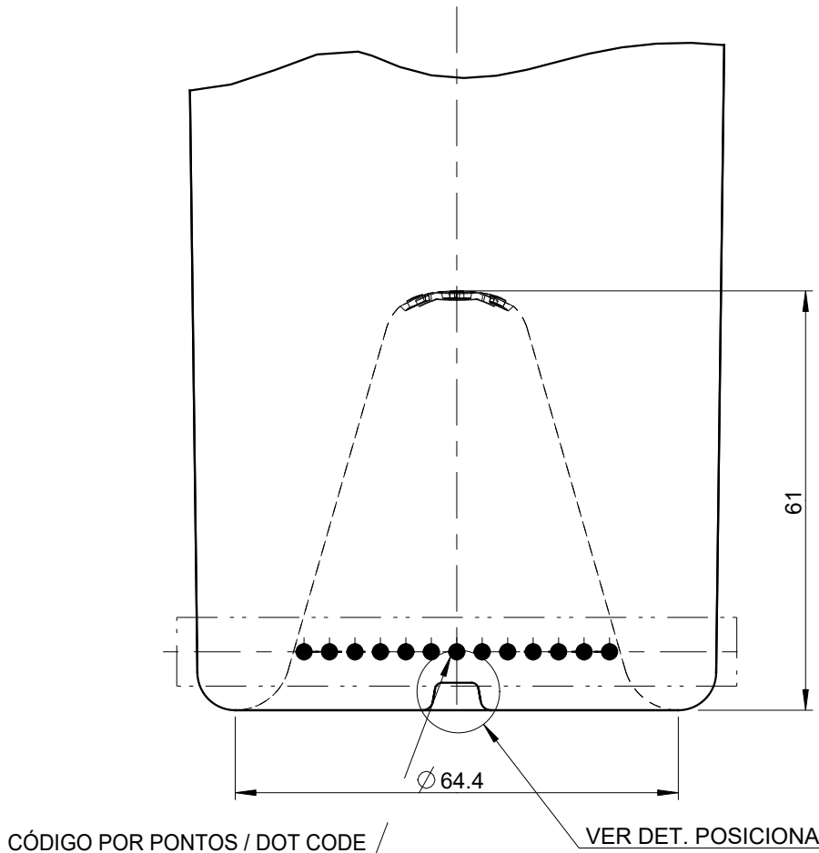
VISTA POSTERIOR / BACK VIEW
