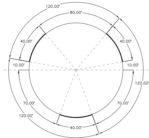
SECCIÓN A-A UBICACIÓN DE GRABADOS EQUIDISTANTES A 120° (UNO AL FRENTE, DOS ATRAS) ESC. 1:1
